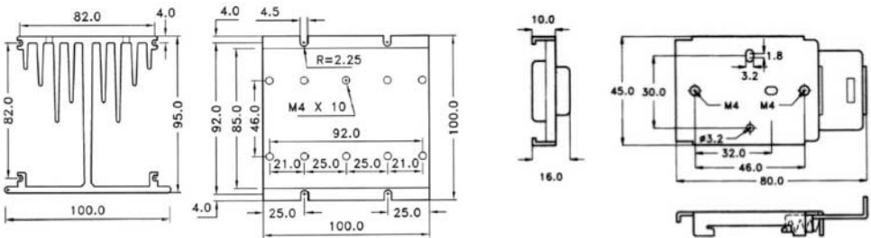
TSR-100 или HS-100: Радиаторы для трехфазных реле
