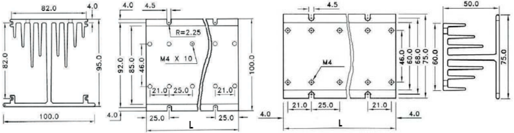
HS-□□□: Радиаторы для реле стандартного типа
