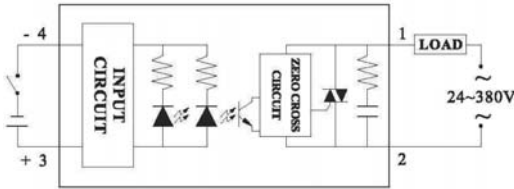
DC-AC тип
