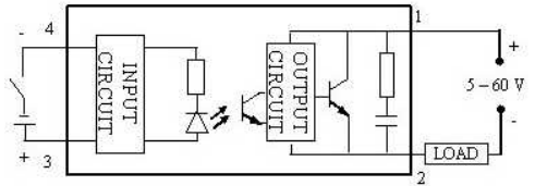
DC-DC тип
